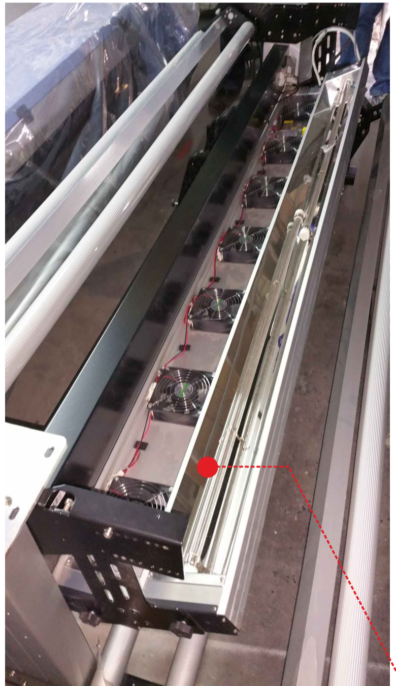
baterie uscare IR si ventilatoare
